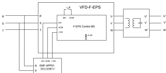
图 1 系统连接示意图
